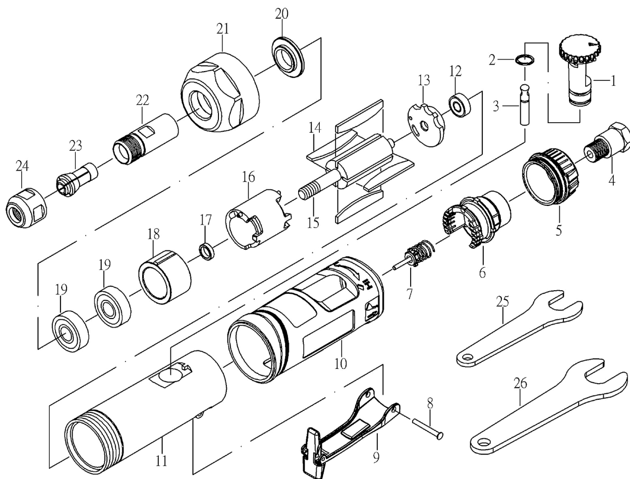
MRA グラインダ MRA-PG35120Ae 分解図
