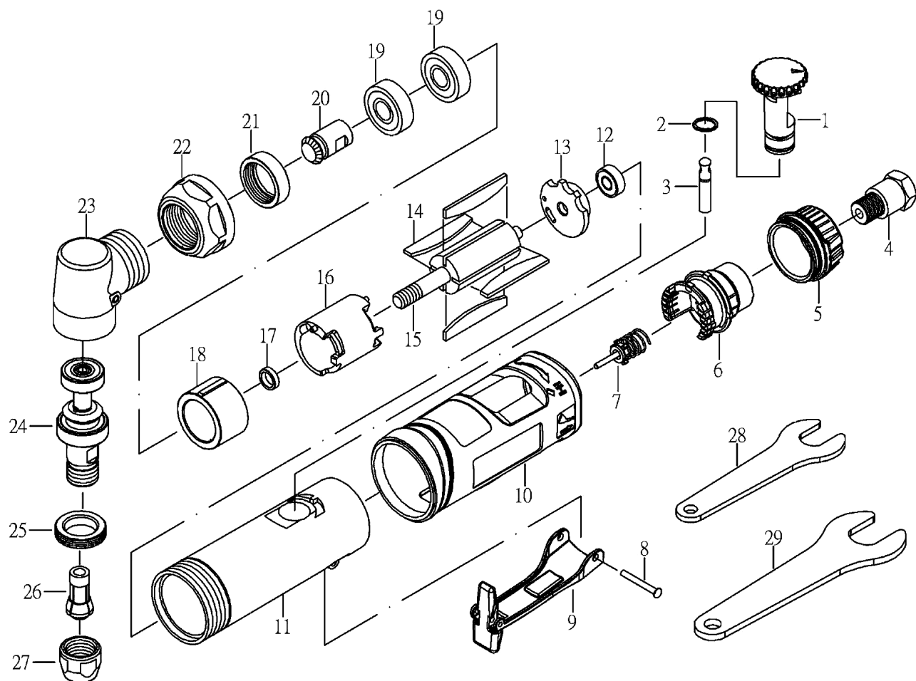
MRA グラインダ MRA-PG35125e 分解図
