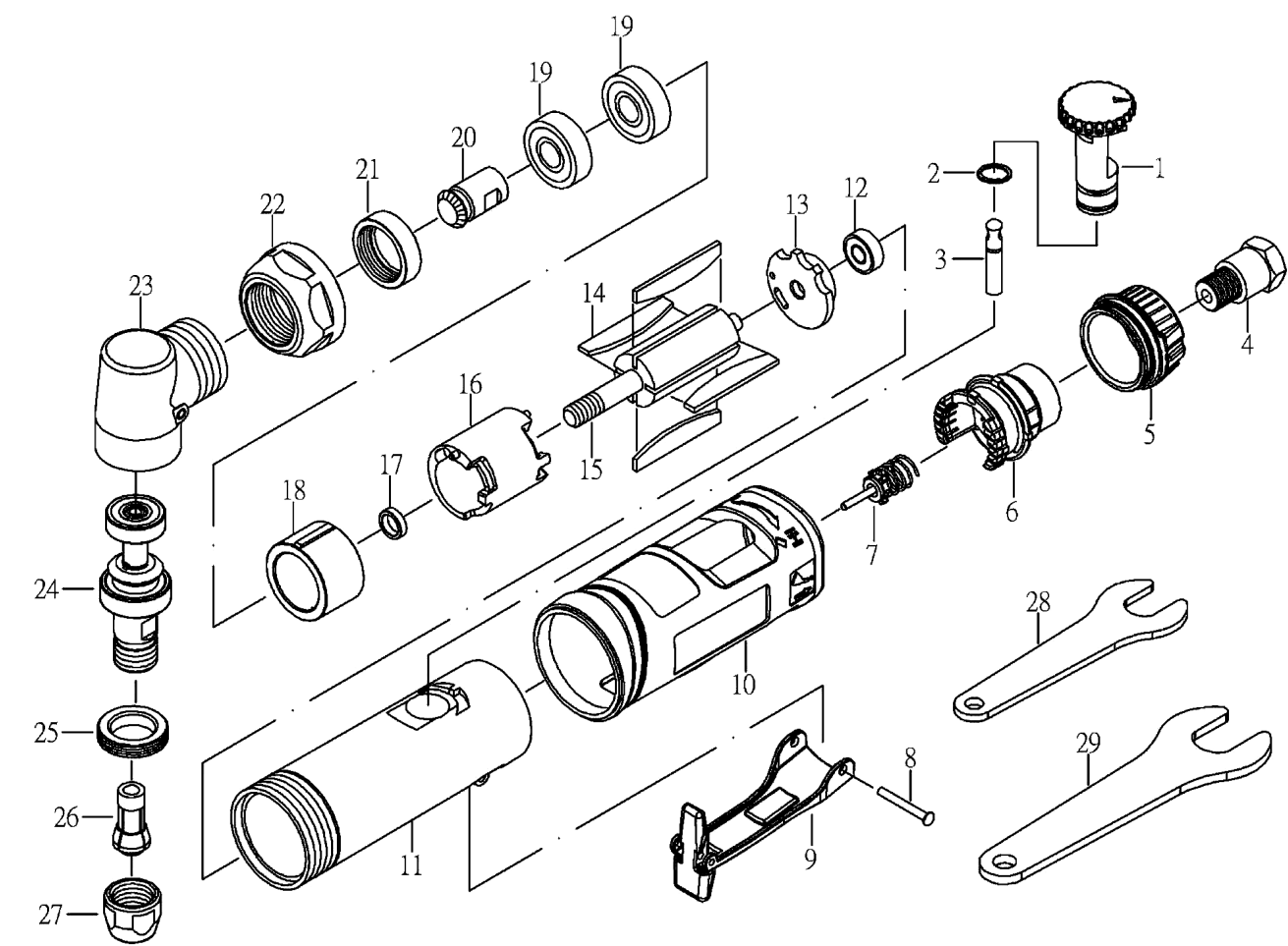
MRA グラインダ MRA-PG35125e 分解図
