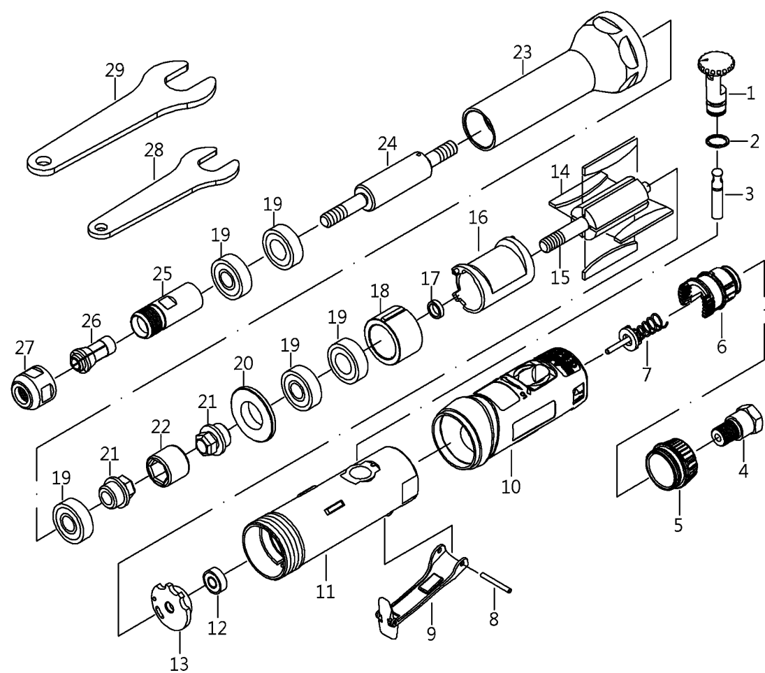
MRA グラインダ MRA-PG50200Le 分解図
