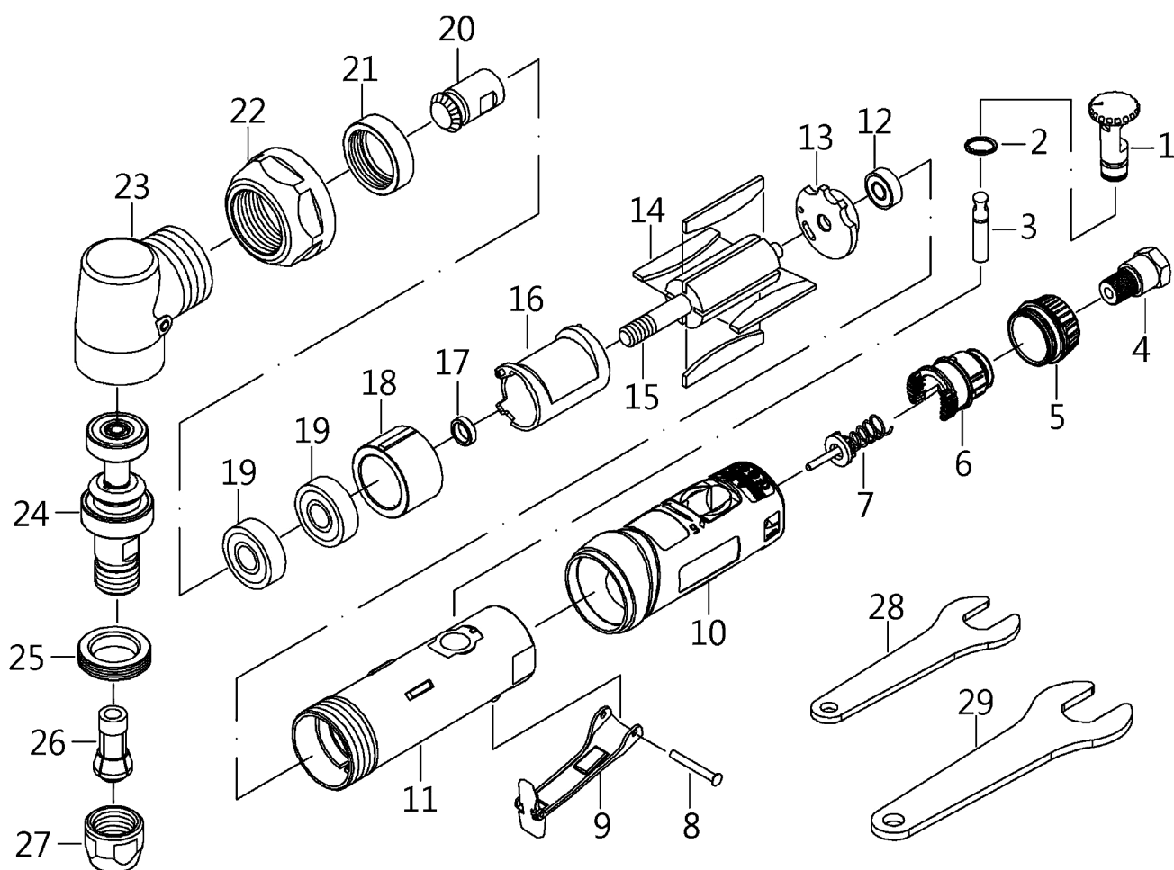
MRA グラインダ MRA-PG50210LSe 分解図
