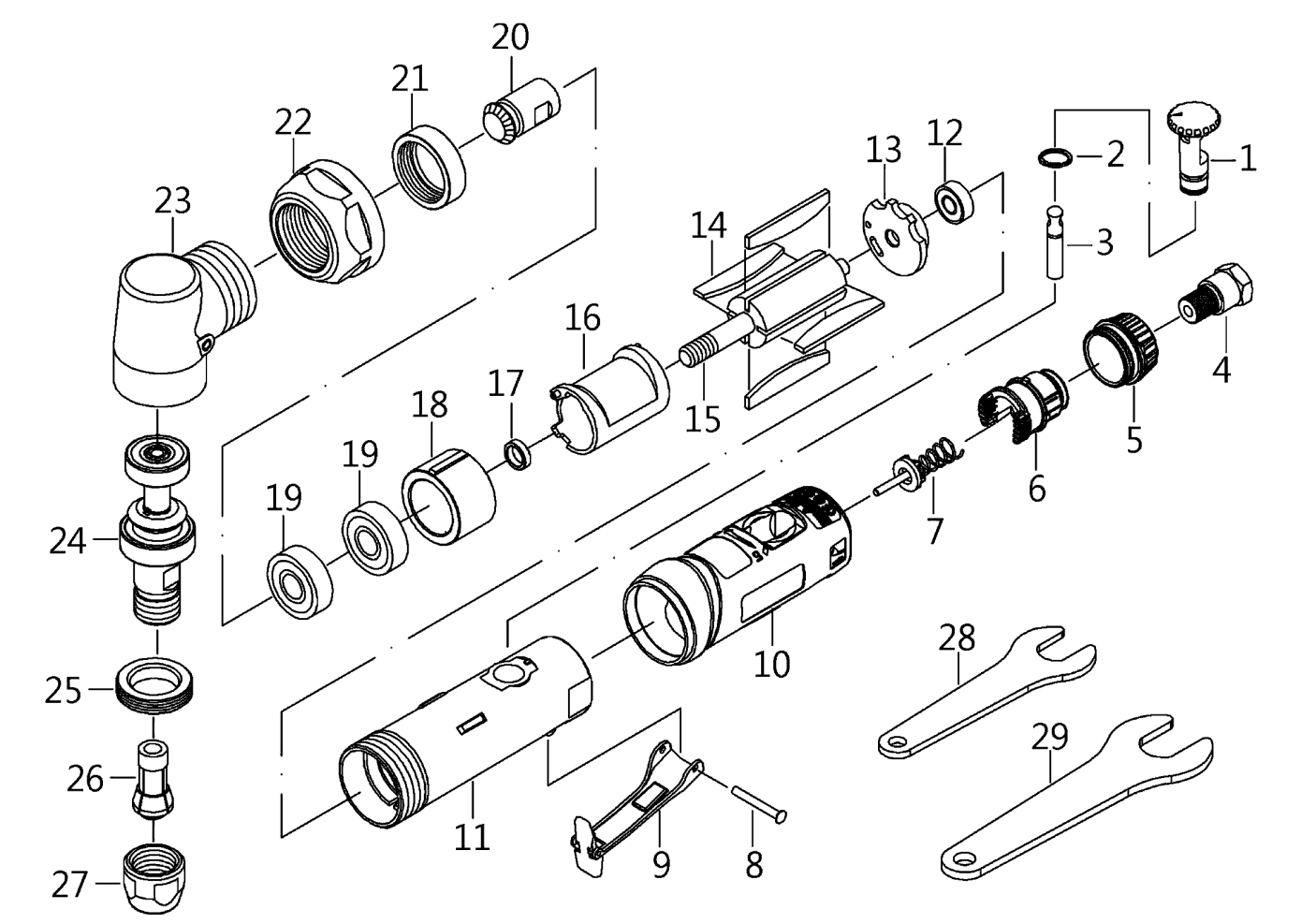
MRA グラインダ MRA-PG50210LSe 分解図
