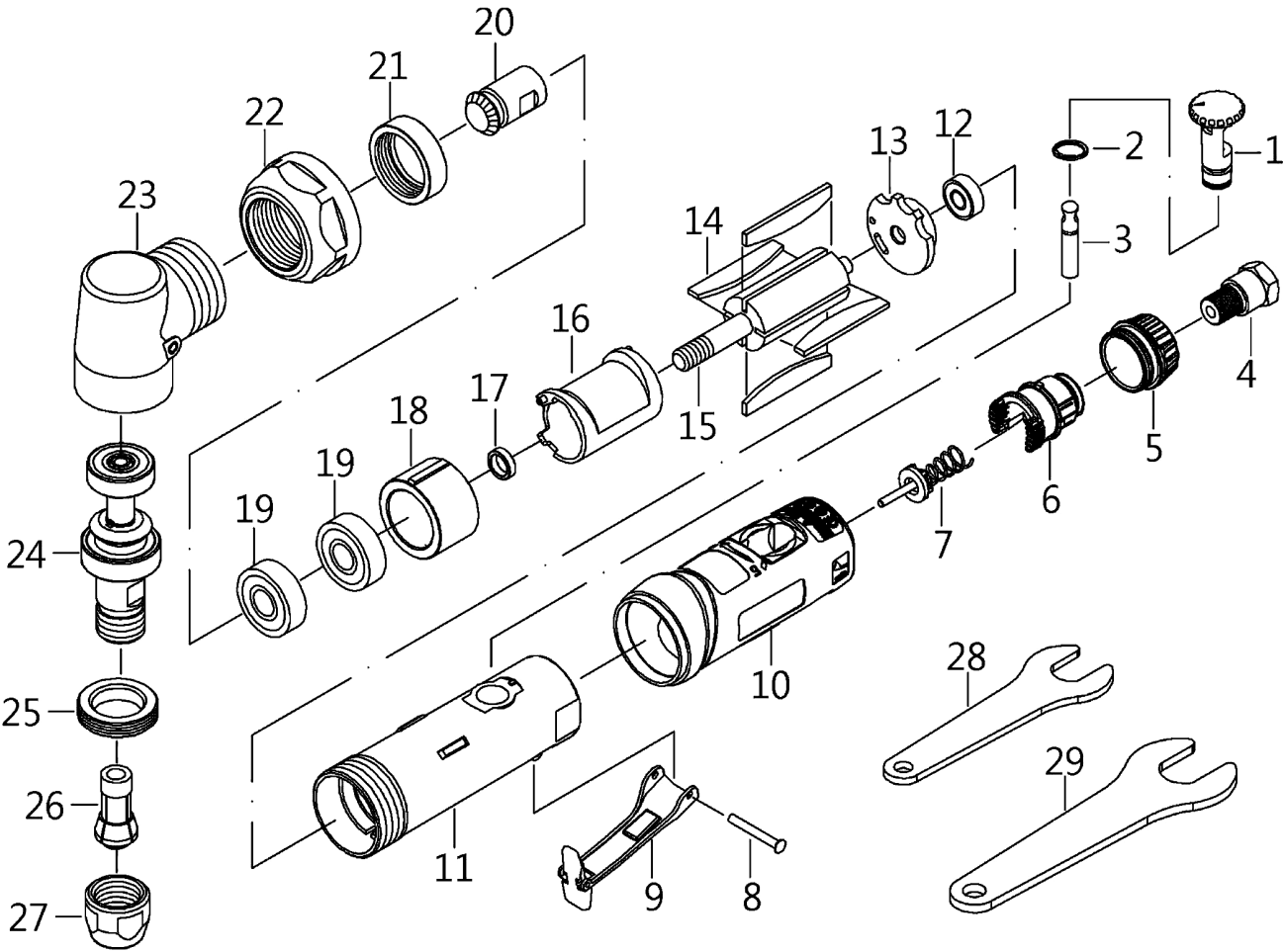
MRA グラインダ MRA-PG50210e 分解図
