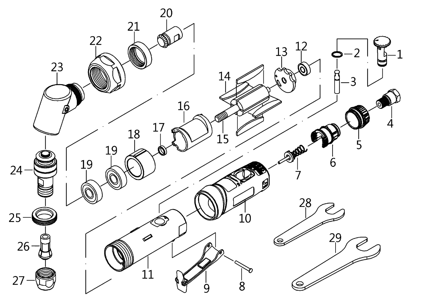
MRA グラインダ MRA-PG502115e 分解図
