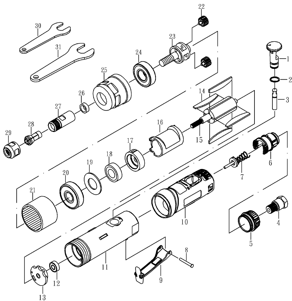
MRA グラインダ MRA-PG50265e 分解図
