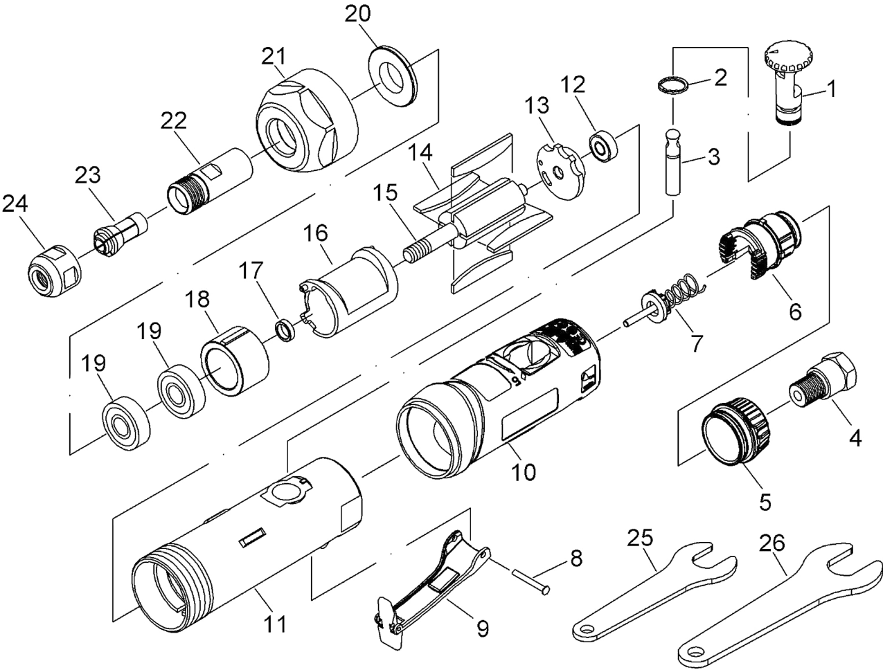
MRA グラインダ MRA-PG50200e 分解図
