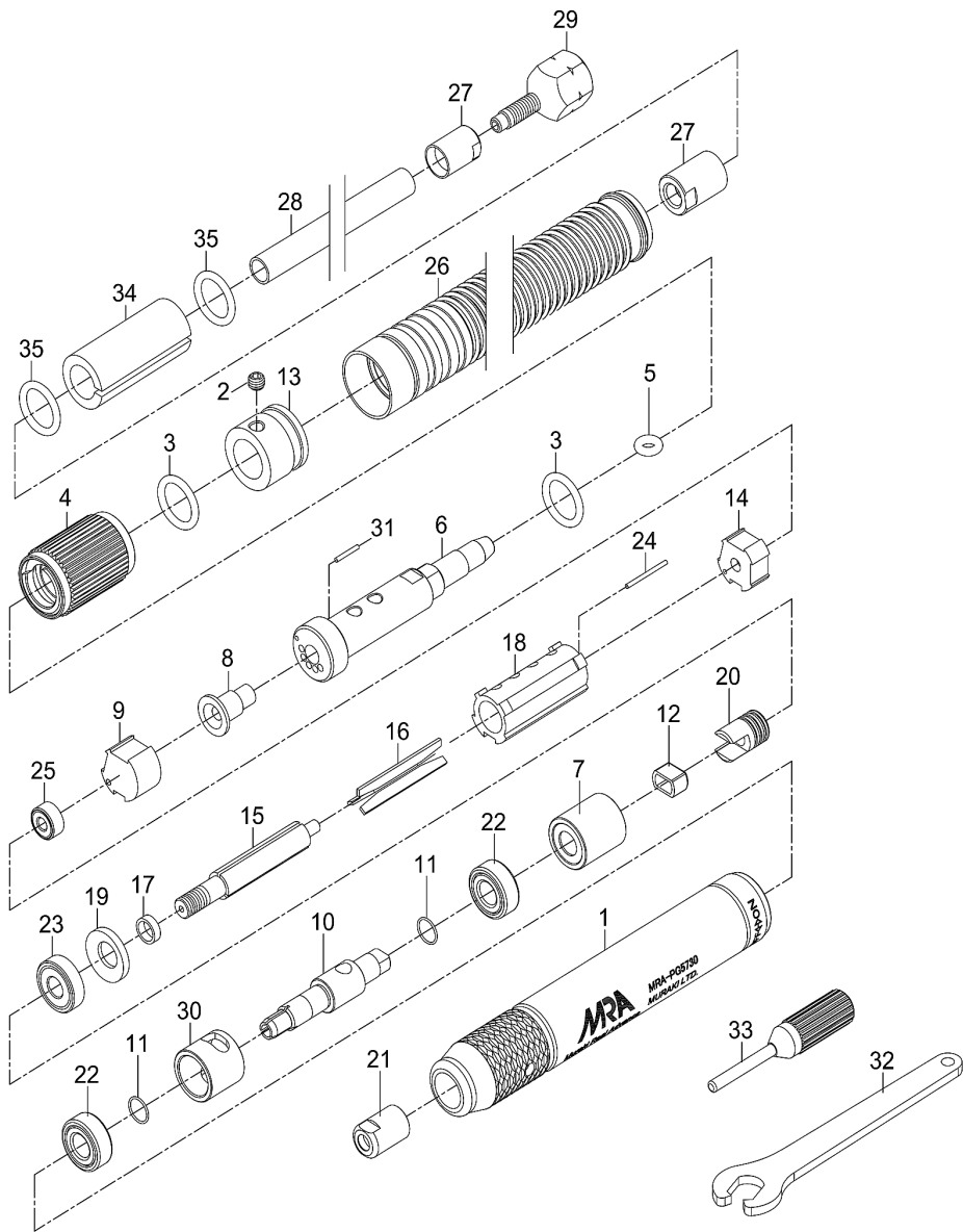
MRA グラインダ MRA-PG5730 分解図
